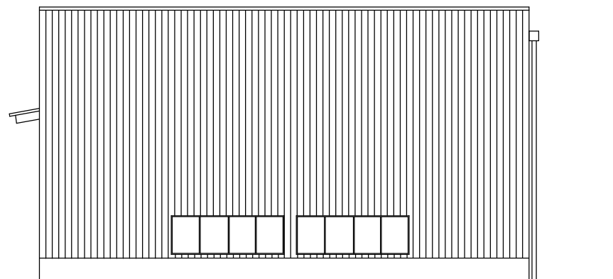
北 立面図
