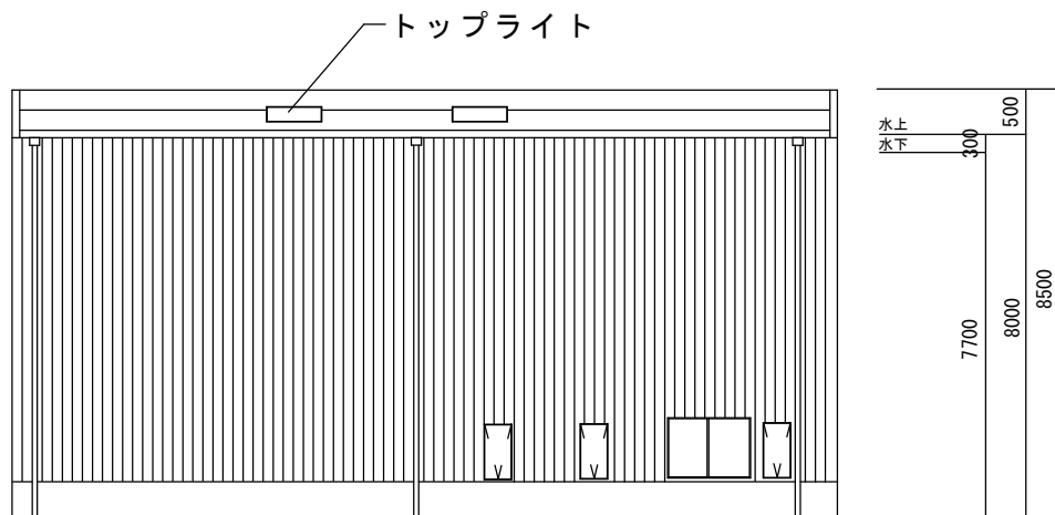
西 立面図
